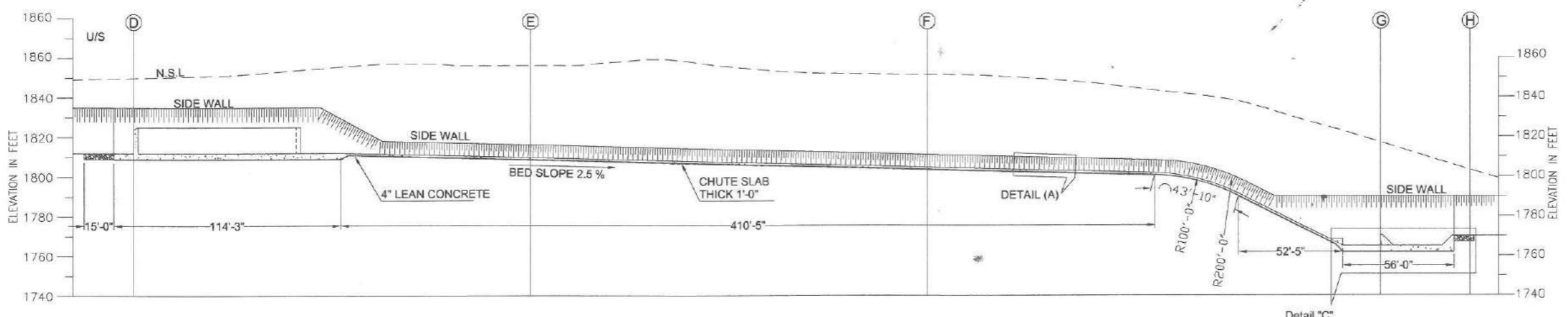
SECTION A-A
