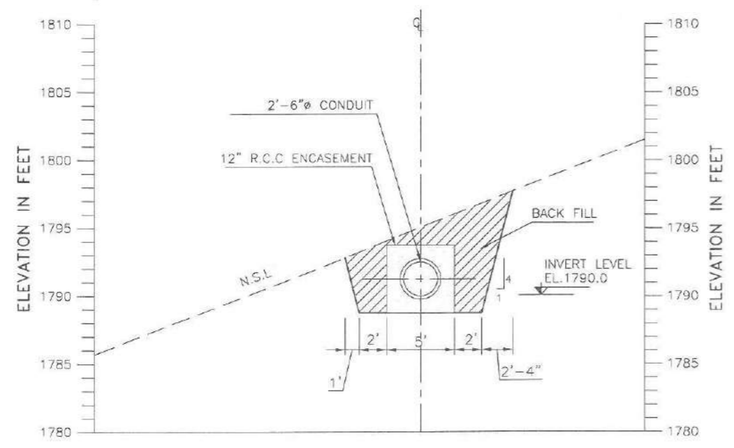
SECTION D-D
