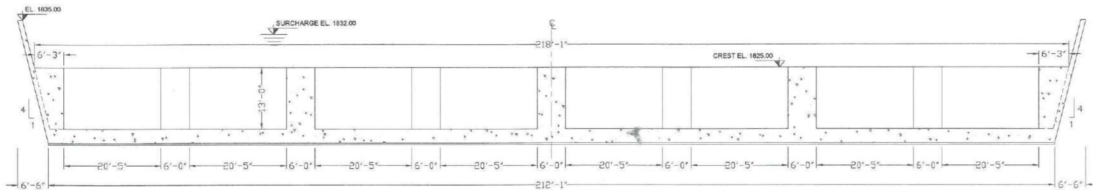
SECTION A-A
