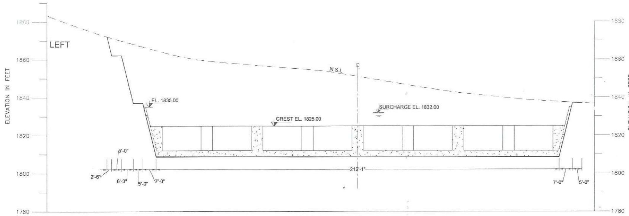
SECTION D-D
